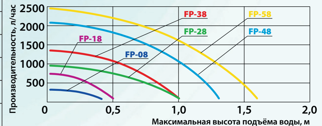
График производительности насосов FP-*8
